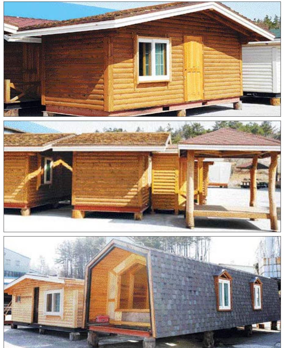
이동식 통나무집의 여러 형태. 위로부터 5평형, 방갈로형, 북층형 구조.
