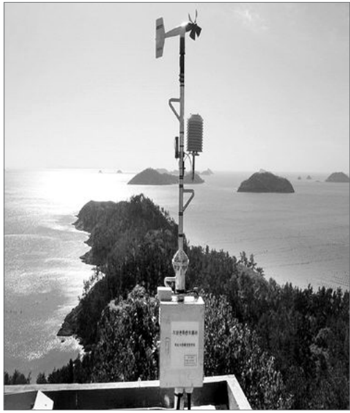
상신호표지에서 파랑, 조류, 수온, 풍향, 풍속, 기온, 습도, 기압 등을 자동 측정해 센터인 진도항로표지 종합관리소로 보내면 센터에서 이를 종합해 전송하게 된다.
