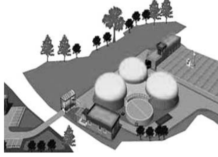
남원 가축분뇨 공동자원화 시설 조감도.
