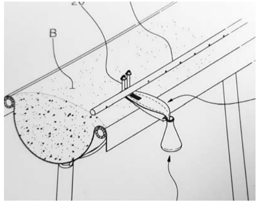
점적관수 배출량 측정장치 개략도.
